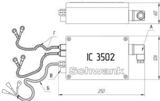
Рисунок 2 Внешний вид. Подключение клапана VR
