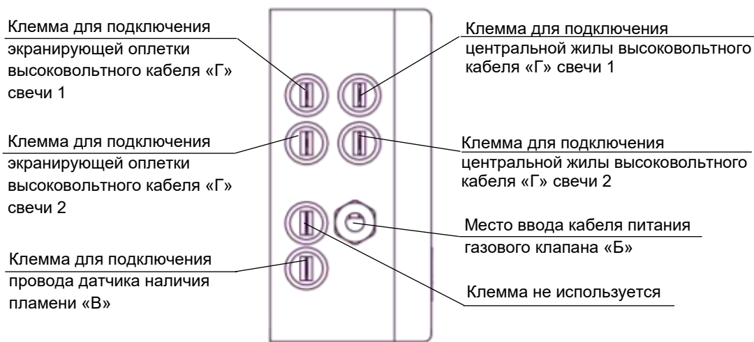
Рисунок 3 Подключение кабелей
